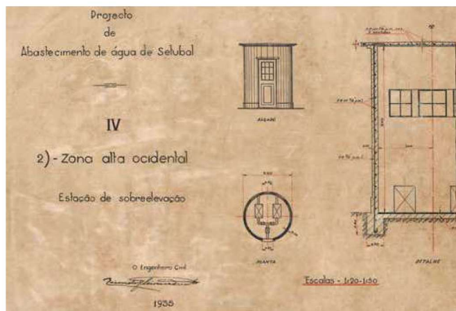
Planta n.º 4 do projeto de abastecimento de água a Setúbal Fonte: Coleção particular de António Pinho. Nota: Autoria do eng.º Ricardo Teixeira Duarte e datada de 1935.
