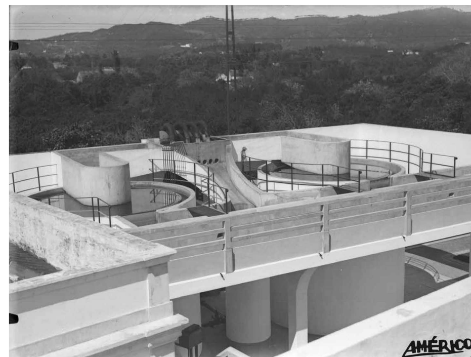
Parte das estruturas da central elevatória de águas (04/04/1940) Fonte: Coleção Américo Ribeiro. Arquivo Fotográfico Américo Ribeiro. PT/AFAMR/AMR-989.
